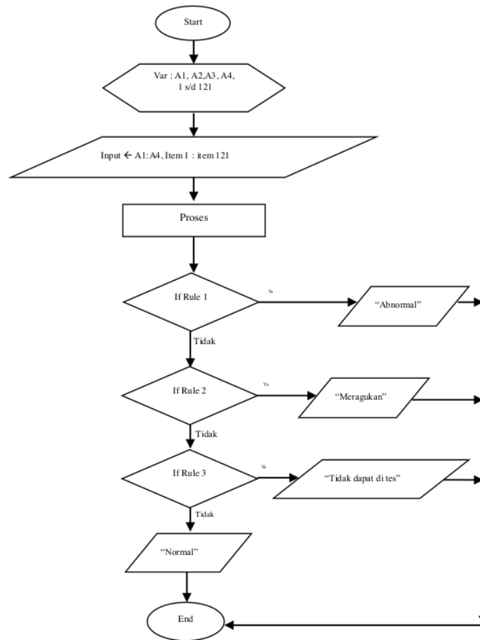
Gambar 6. Flowchart Model Identifikasi Monitoring Perkembangan Anak
