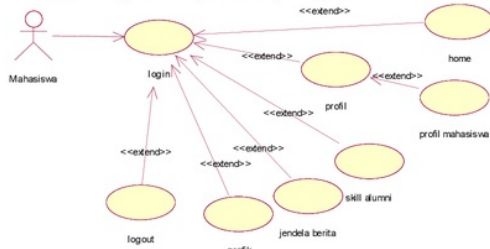
Gambar 2.4 Use Case Diagram Mahasiswa
