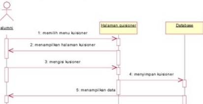
Gambar 2.9 Sequence Diagram mengakses kuisioner
