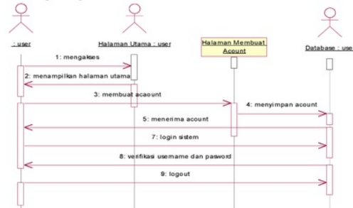
Gambar 2.6: User mendaftar di sistem
