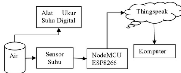
Gambar 3. Perancangan Karakterisasi dan Kalibrasi Sensor LM 35
