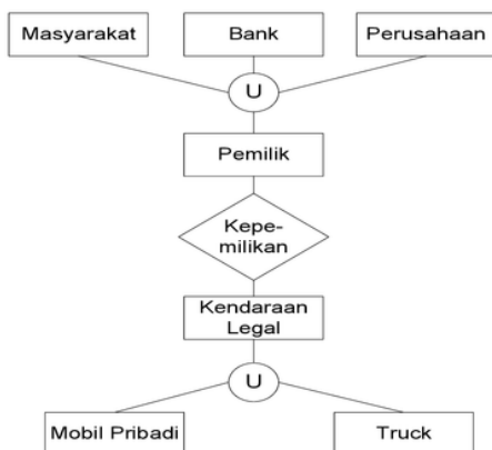
Gambar 4. EER-D Notasi untuk categorization (adaptasi dari [10])
