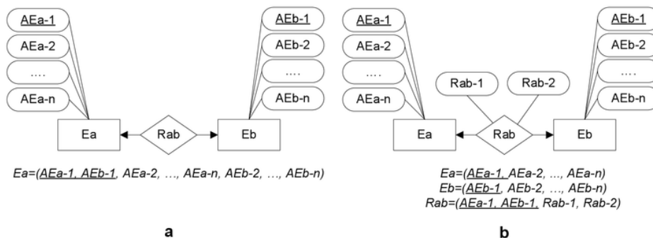
Gambar 5. Transformasi ER-D derajat 1-to-1 menjadi skema relasional
