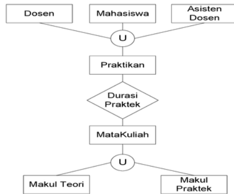
Gambar 12. Kategorisasi dengan gabungan beberapa entitas
