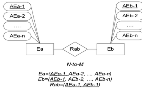
Gambar 7. Transformasi ER-D derajat N-to-M menjadi skema relasional
