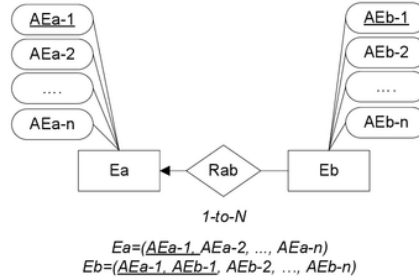
Gambar 6. Transformasi ER-D derajat 1-to-N menjadi skema relasional
