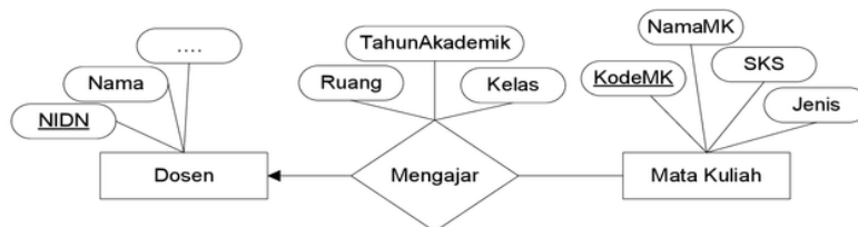
Gambar 2. ER-D sederhana dengan 2 entitas
