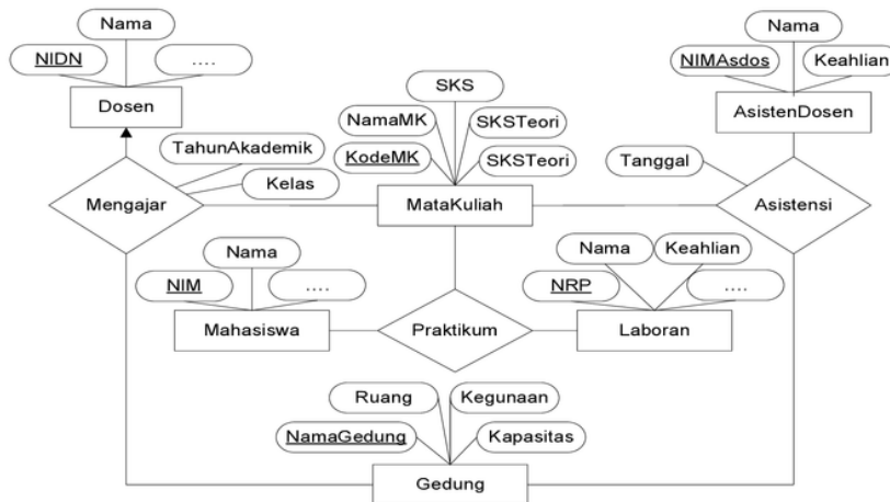
Gambar 8. ER-D sistem asistensi
