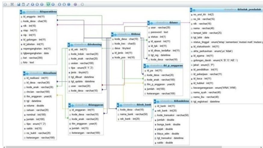
Gambar 5. Relasi tabel
