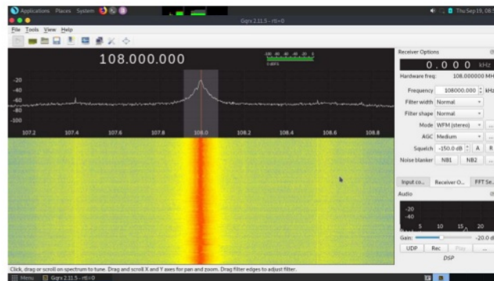
Gambar 5. Pengujian Pemancar FM pada frekuensi 88.8 MHz
