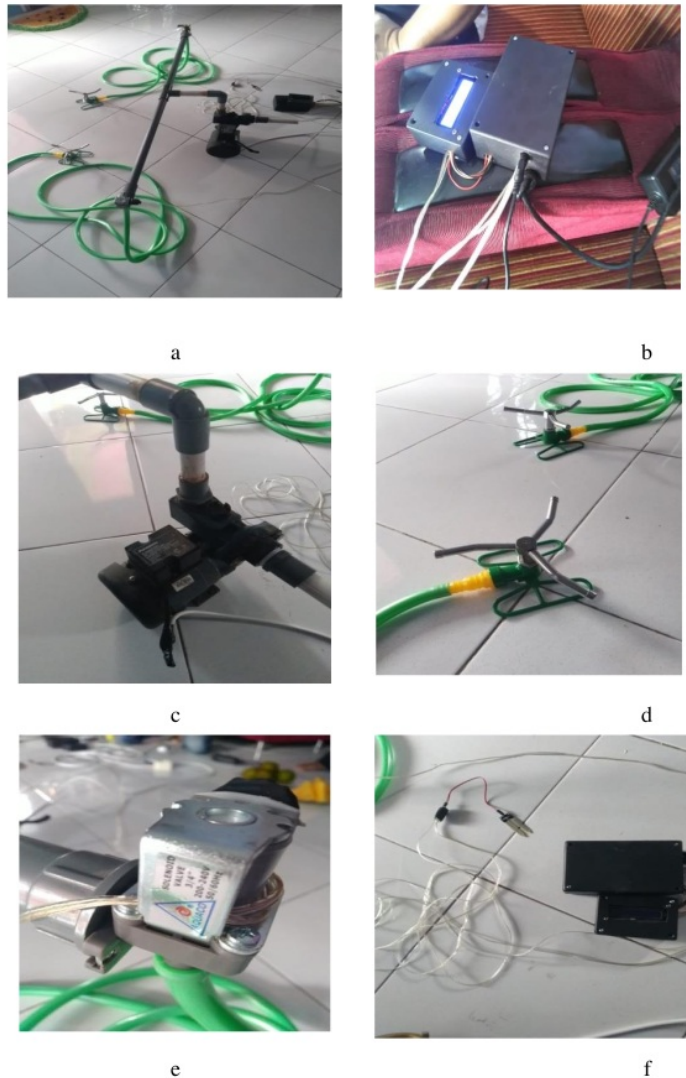
Gambar 3. Alat penyiram tanaman bawang merah (a) Sistem secara keseluruhan, (b) Mikrokontroler ,(c) Pompa Air, (d) Sprinkler, dan (e) Selenoid Valve, dan (f) Sensor Kelembaban
