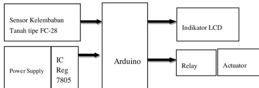
Gambar 1. Diagram blok sistem penyiram tanaman bawang
