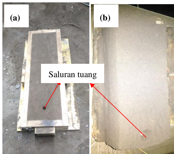
Gambar 4. Cetakan yang digunakan (a) sand casting/SC (b) investment casting/IC
