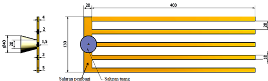
Gambar 3. Desain cetakan untuk uji fluiditas
