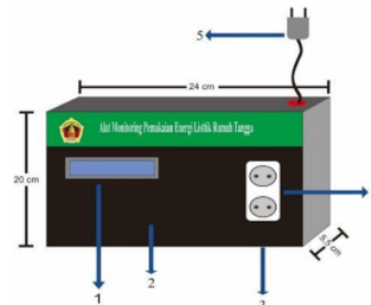
Gambar 4. Desain Perancangan Alat
