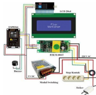
Gambar 3. Perancangan Wiring Pemakaian energi Listrik
