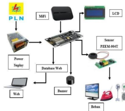
Gambar 2. Perancangan Hardware
