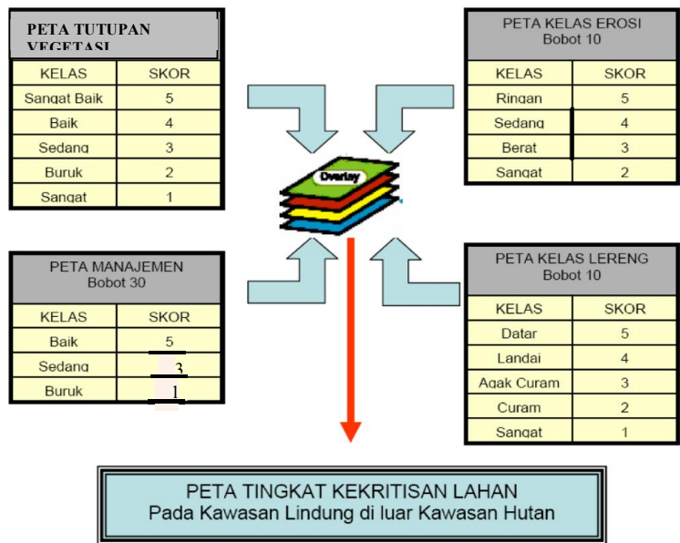
Gambar 4. Kriteria & prosedur penetapan lahan kritis kawasan lindung di luar kawasan hutan
