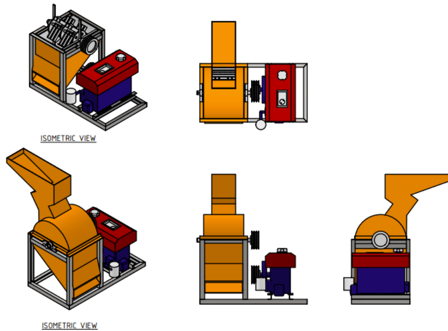
Gambar Sketsa Prototype Mesin Penggiling Limbah Gerabah Pecahan Gerabah, Genteng, Batu Bata dan Kaca - 3 D
