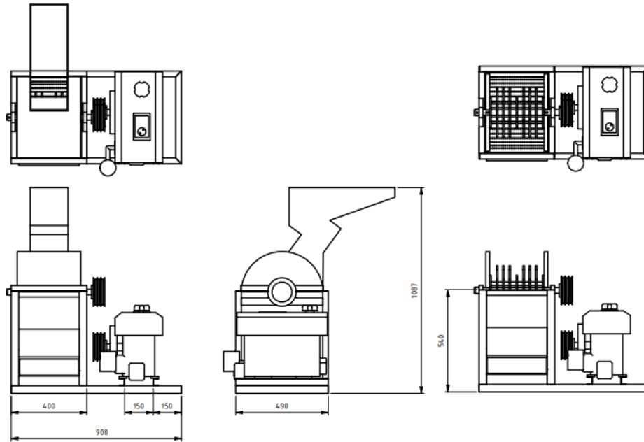
Gambar Sketsa Prototype Mesin Penggiling Limbah Gerabah Pecahan Gerabah, Genteng, Batu Bata dan Kaca - 2 D
