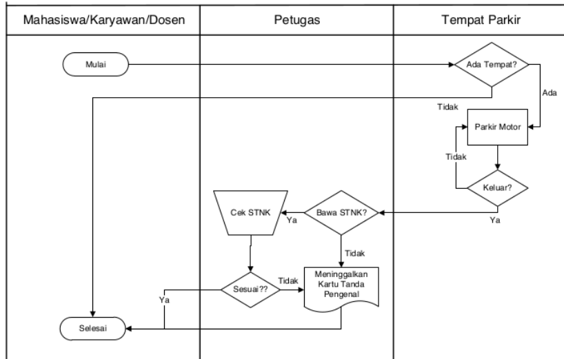
Gambar 3. FOD Sistem parkir di Universitas Muria Kudus
