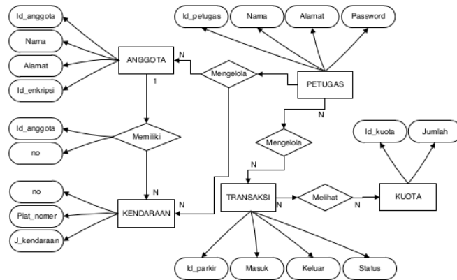
Gambar 6. ERD parkir di Universitas Muria Kudus dengan menggunakan enkripsi data dan teknologi Barcode
