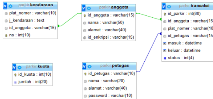
Gambar 7. Relasi antar tabel
