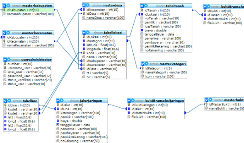
Gambar 8. Relasi Antar tabel
