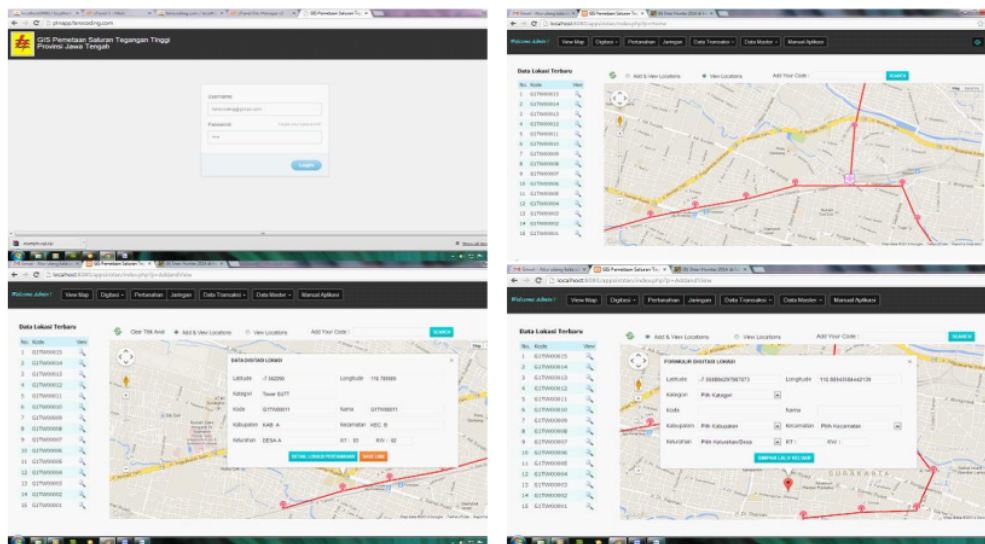
Gambar 9. Capture Aplikasi
