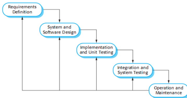
Gambar 4 Metodologi Waterfall
