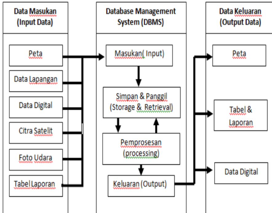
Gambar 2 Uraian subsistem-sistem SIG.
