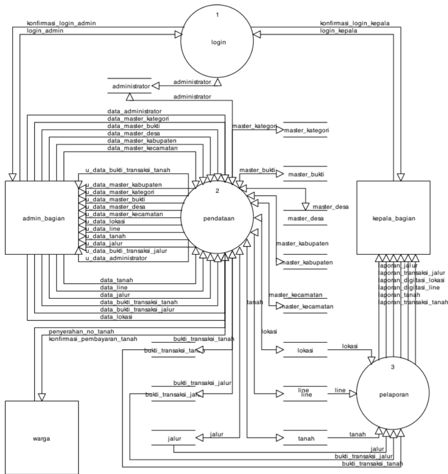
Gambar 6 DFD Level 0 Pendataan Pengarsipan Aset PLN
