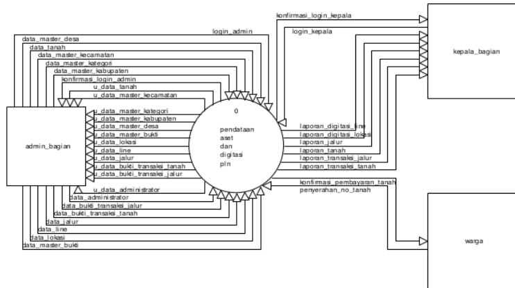
Gambar.5 Context Diagram Pendataan Pengarsipan Aset PLN
