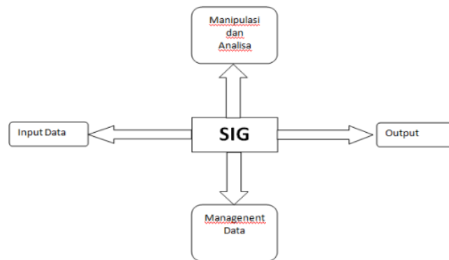
Gambar 1 Subsistem-subsistem SIG
