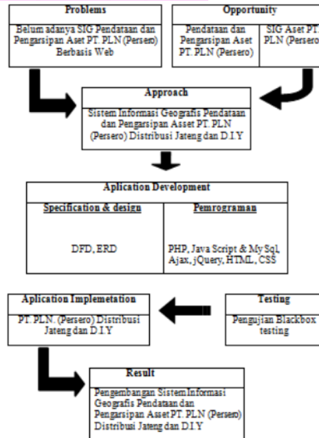
Gambar 3 Kerangka Pemikiran
