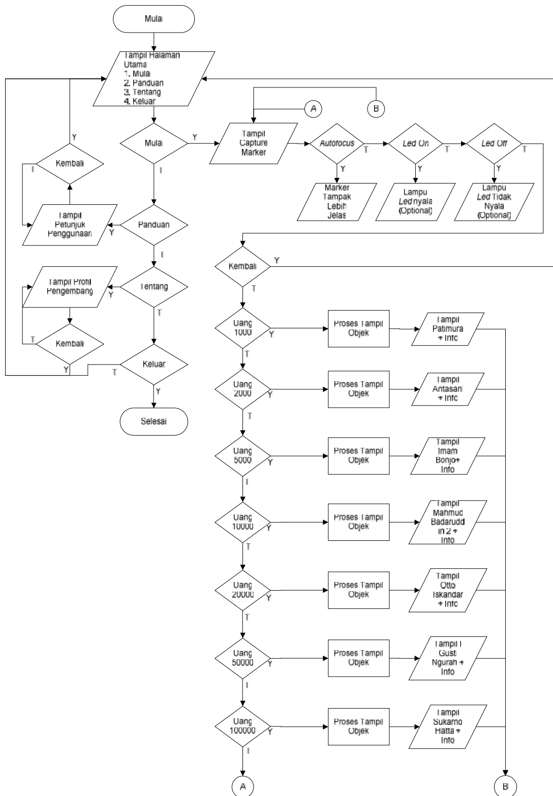
Gambar 2. Flowchart Aplikasi
