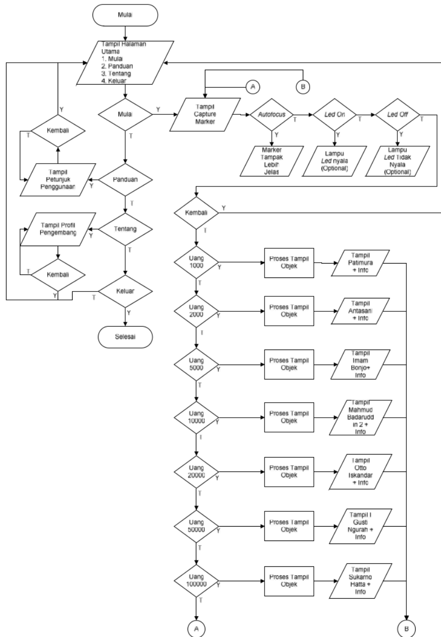
Gambar 2. Flowchart Aplikasi
