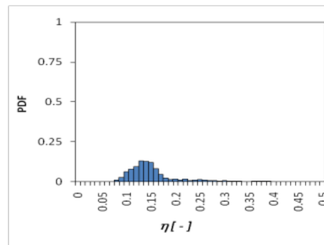
Gambar 13. Contoh PDF Pola Aliran Pseudo-Slug ( J_L = 0,092 m/s dan J_G = 3.77 m/s)
