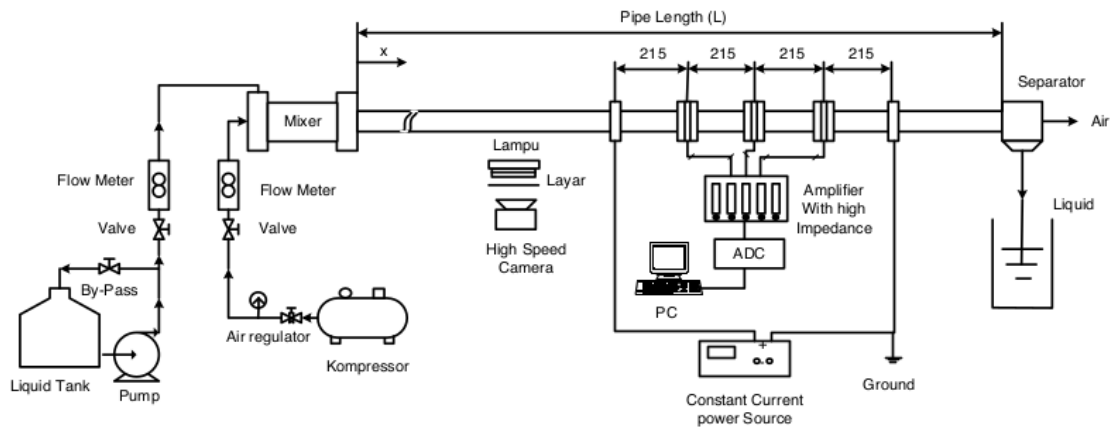
Gambar 1. Skema Diagram Peralatan
