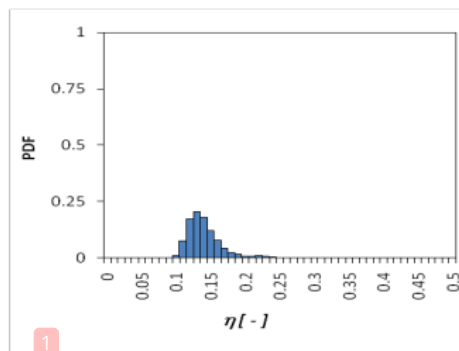
Gambar 10. Contoh PDF Aliran Stratified Wavy + Roll ( J_L = 0,047 m/s dan J_G = 3.77 m/s)
