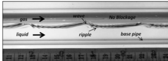
Gambar 5. Visualisasi Aliran Stratified Wavy + Ripple ( J_L = 0,092 m/s dan J_G = 1,02 m/s)
