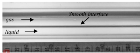
Gambar 2. Contoh Visualisasi Aliran Stratified Smooth ( J_L = 0,016 m/s dan J_G = 1,02 m/s)
