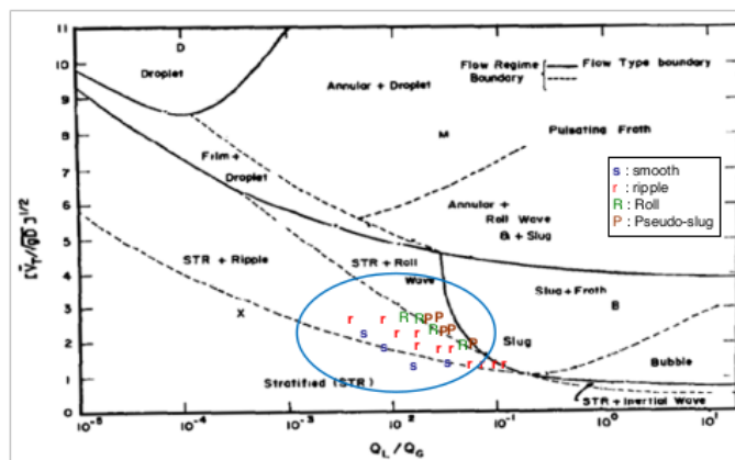
Gambar 15. Perbandingan Data Penelitian Dengan Peta Pola Aliran Spedding dan Nguyen (1979)
