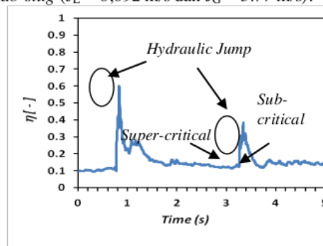
Gambar 12. Contoh Liquid Hold-Up Pola Aliran Pseudo-Slug ( J_L = 0,092 m/s dan J_G = 3.77 m/s)
