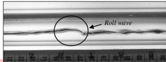
Gambar 8. Contoh Visualisasi Aliran Stratified Wavy + Roll ( J_L = 0,047 m/s dan J_G = 3.77 m/s)
