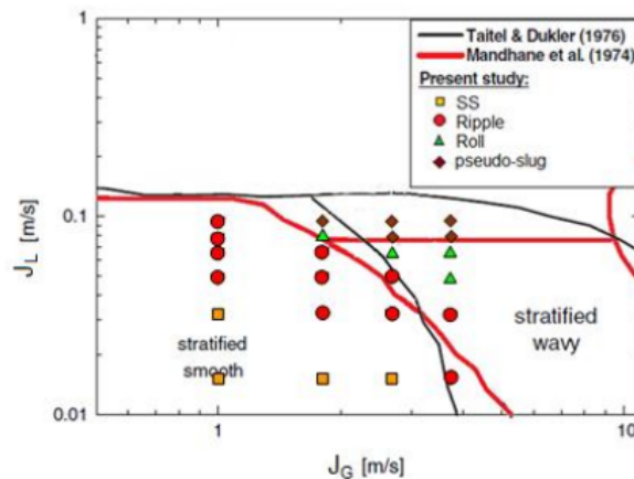
Gambar 14. Perbandingan Data Penelitian Dengan Peta Pola Aliran Mandhane (1974) Serta Taitel Dan Dukler (1976)
