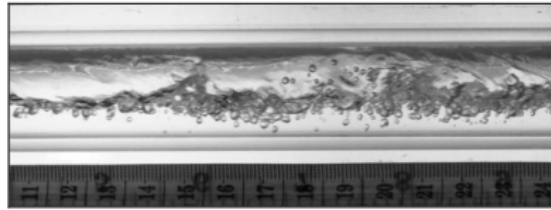
Gambar 11. Contoh Visualisasi Pola Aliran Pseudo-Slug ( J_L = 0,092 m/s dan J_G = 3.77 m/s)
