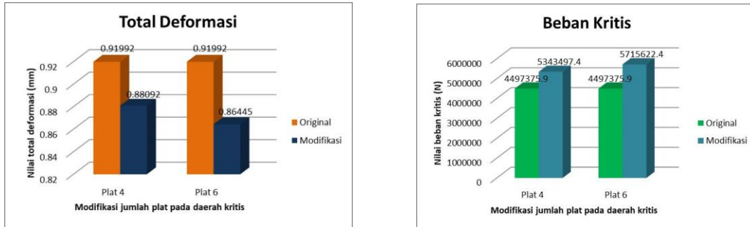
(a) (b) Gambar 19. Grafik perbandingan modifikasi jumlah plat (a) Total deformasi (b) Beban kritis
