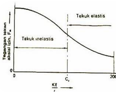
Gambar 6. Hubungan tegangan kritis dan rasio kelangsingan (KL/r)
