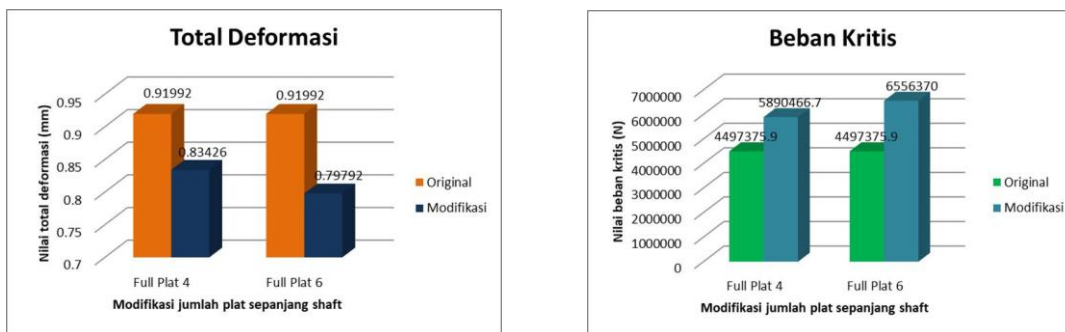
(a) (b) Gambar 20. Grafik perbandingan modifikasi jumlah full plat (a) Total deformasi (b) Beban kritis
