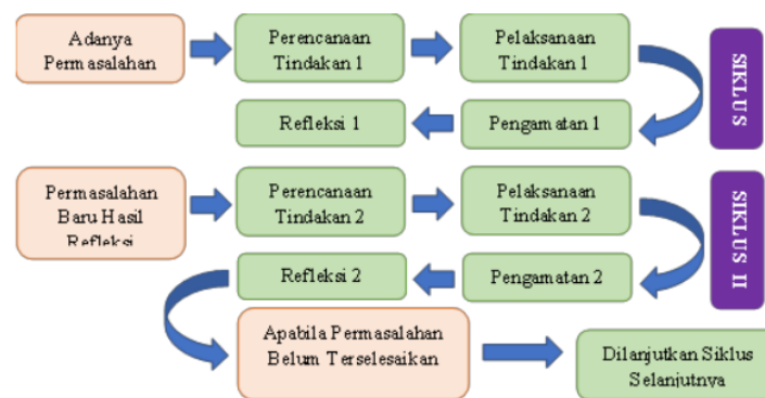
Gambar 1. Desain Penelitian
