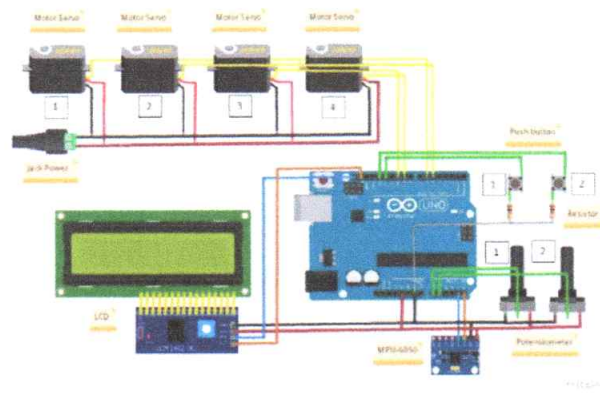
Gambar 3. Skema Perancangan Alat
