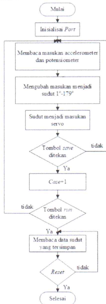
Gambar 2. Perancangan Software
