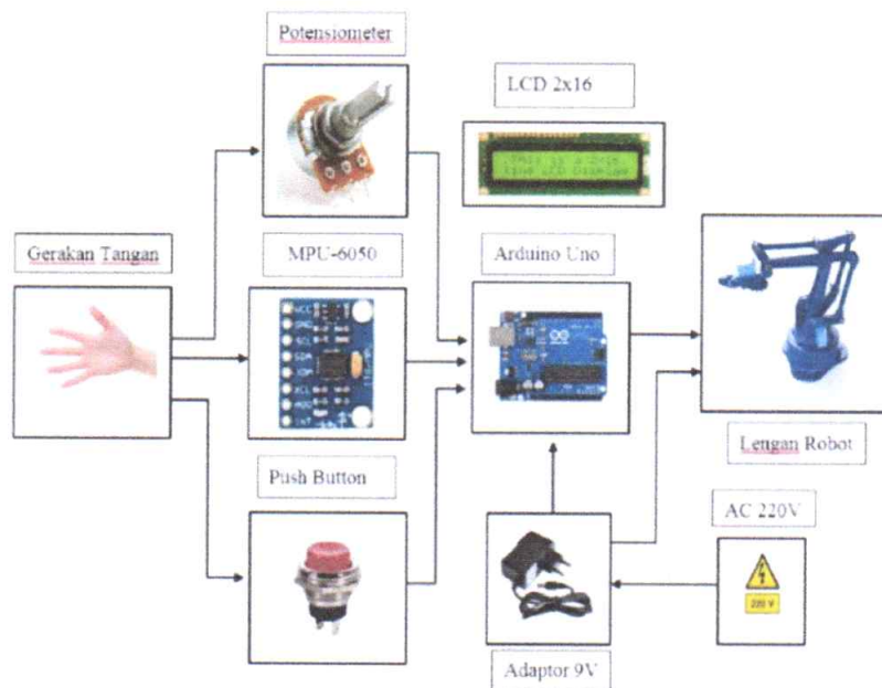
Gambar 1. Perancangan Hardware
