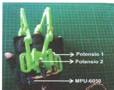
Gambar 7. Hasil Perakitan Sarung Tangan
