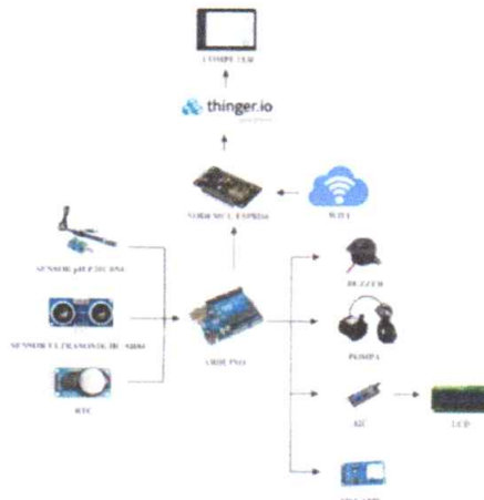
Gambar 2 Perancangan Keseluruhan Hardware
