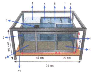
Gambar 4 Perancangan Keseluruhan Sistem Prototipe Tampak Samping Kanan
