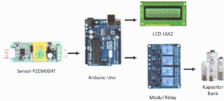
Gambar 3. Desain Skema Alat Koreksi Faktor Daya
