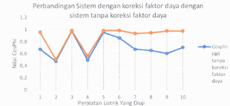
Gambar 7. Perbandingan sistem dengan koreksi faktor daya dan sistem tanpa koreksi faktor daya
