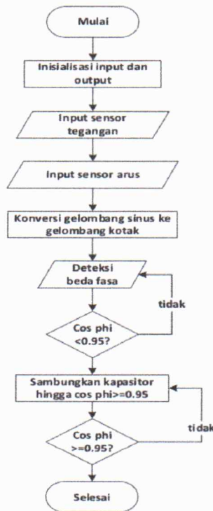
Gambar 4. Diagram Alir Cara Kerja Sistem Koreksi Faktor Daya
