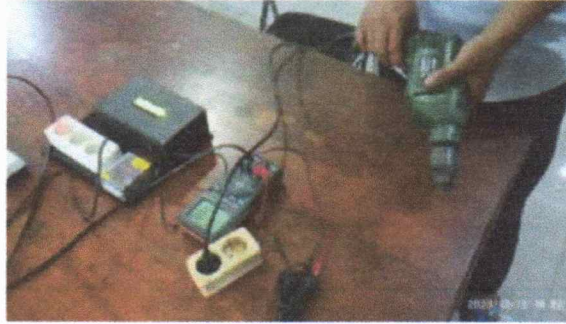
Gambar 6. Proses Pengujian Alat Koreksi Faktor Daya dengan beban handdrill
