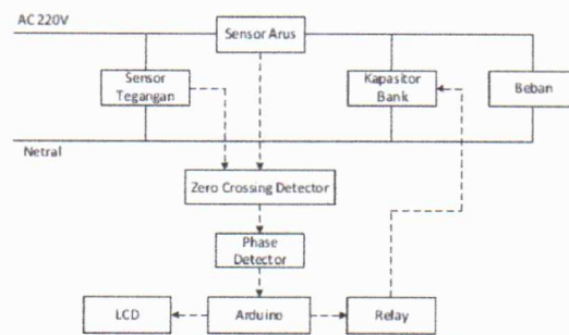
Gambar 2. Diagram Blok Sistem Alat Koreksi Faktor Daya
