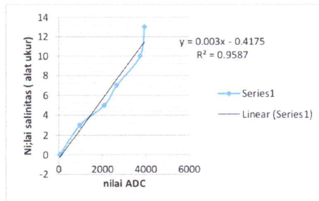
Gambar 2. Grafik Karakterisasi
